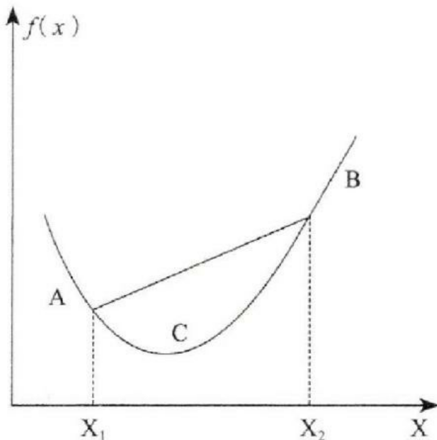
图 2-1 凸函数
