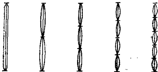
图5. 发音体（弦）的振动图
