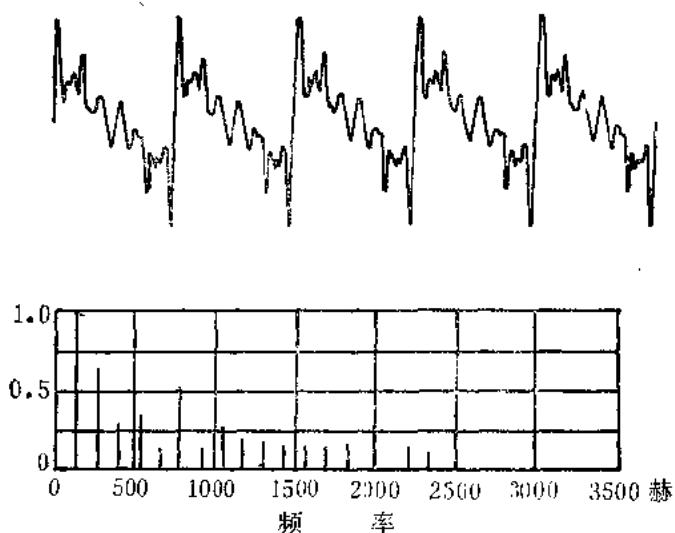
图6. 钢琴音C=128赫的波形记录和声谱图
