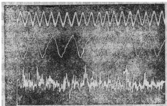
图7. 各种声音振动的记录
