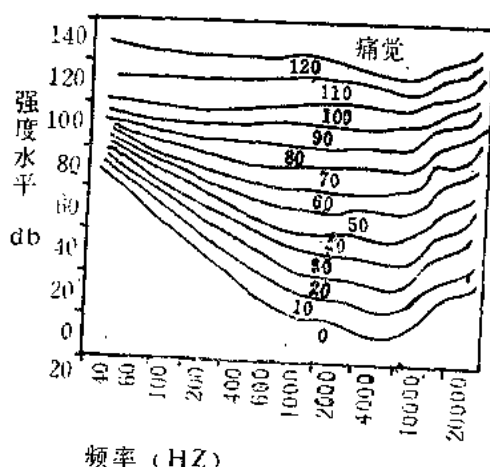
图3. 声音的等响曲线
