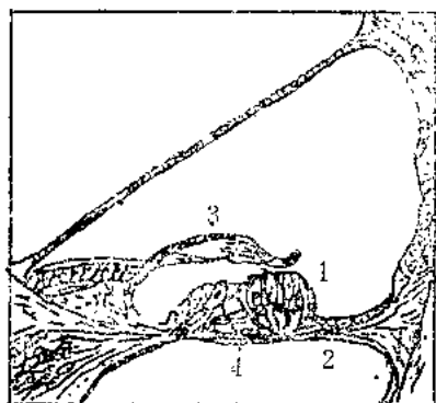
图2. 科蒂氏器官构造的模式图。
