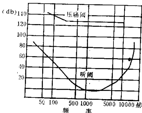
图8. 听觉的阈限曲线
