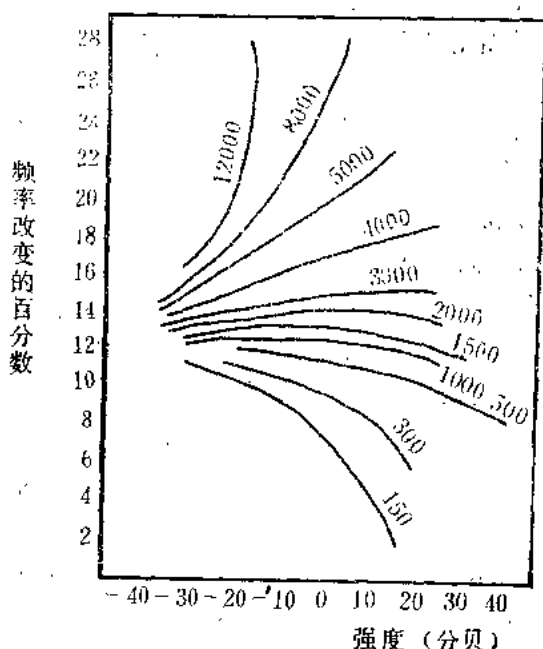
图 4. 音高随强度改变的曲线
