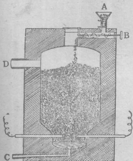
第六十一圖 磷的製造
