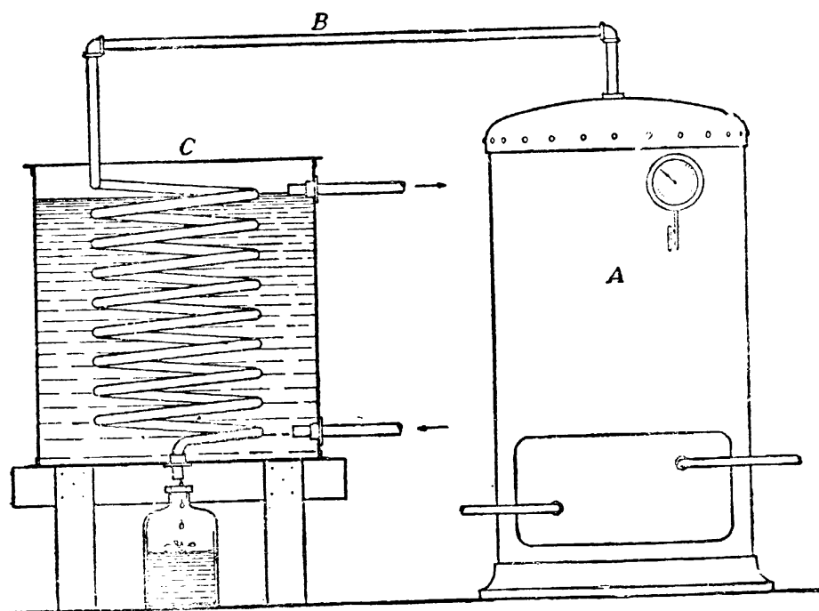
第十八圖 普通用的蒸餾器
