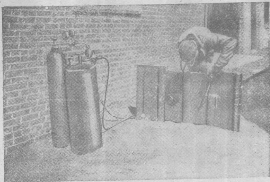
第十三圖 用輕氣與養氣的混合氣體燃燒割取鋼板
