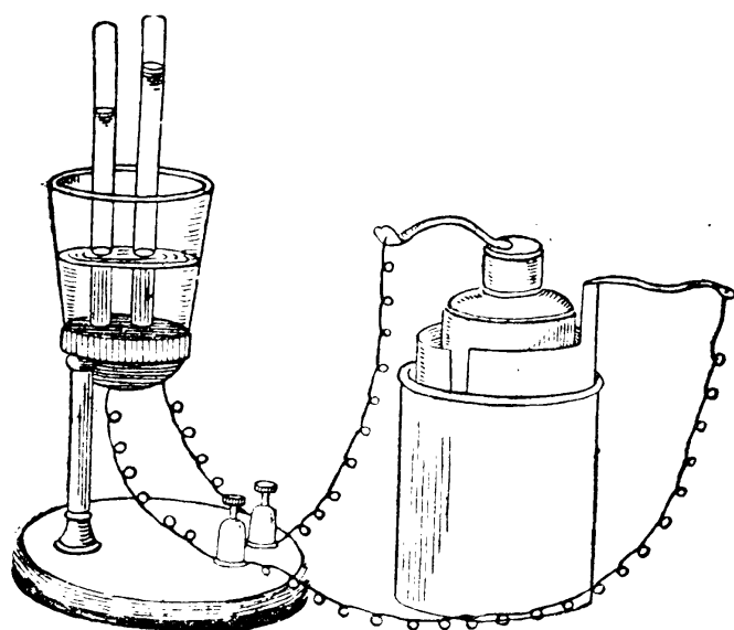
第十九圖 電流分水器
