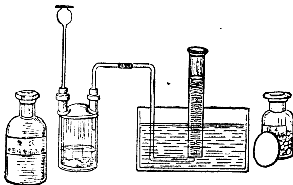
第二十二圖 製輕氣法二
