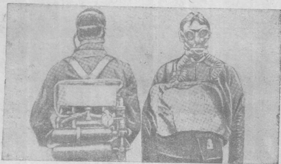
第十二圖 背負壓縮養氣筒的人他的前面右方 繫一皮袋通管於口以便呼出氣體
