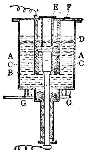
第三十圖 鈉的製造
