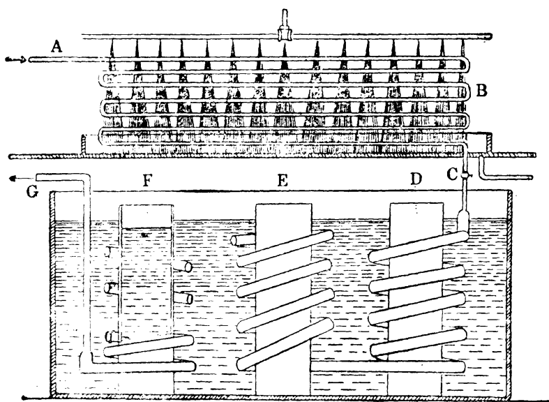
第五十二圖 銨氣製冰機
