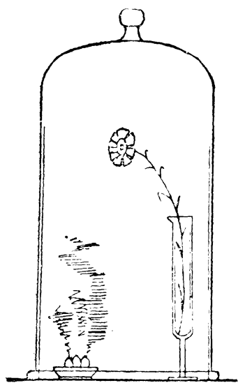
第四十六圖 二氧化硫的漂白作用
