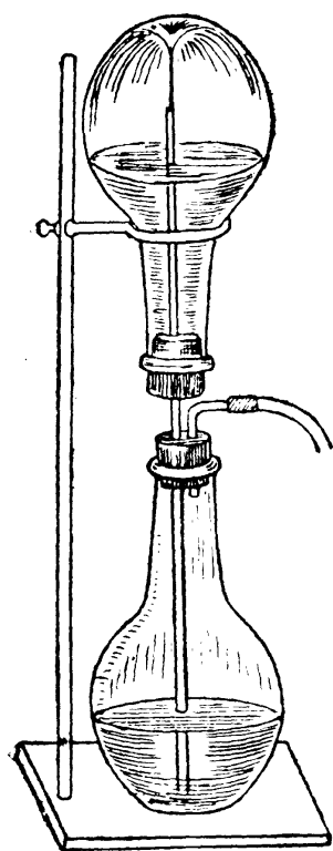
第三十三圖 噴泉
