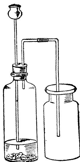
第五十六圖 碳酸氣的製造
