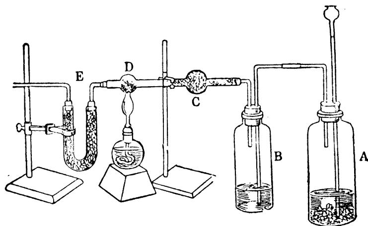
第二十五圖 水的重量組成
