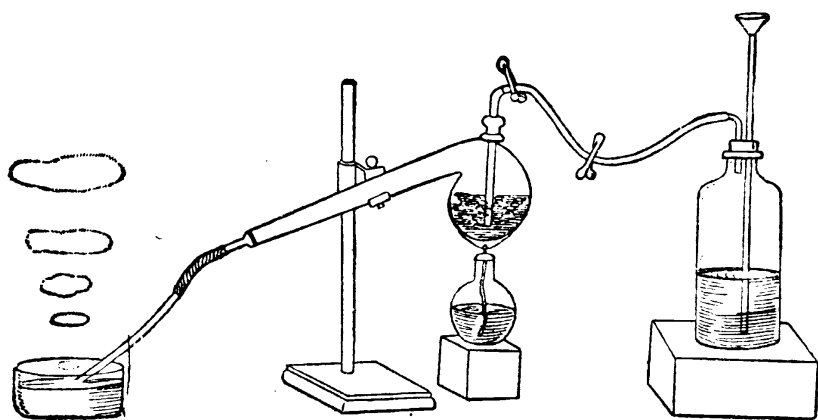
第六十二圖 磷化氫的製造
