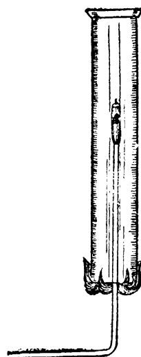
第二十三圖 燭火入輕 氣瓶內
