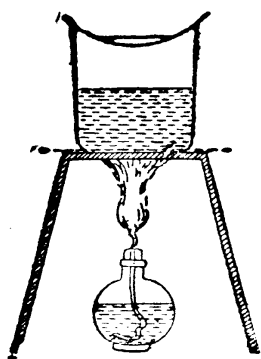
第十五圖 煮沸驗水法
