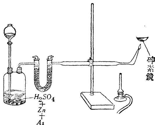
第六十三圖 砷素檢出法
