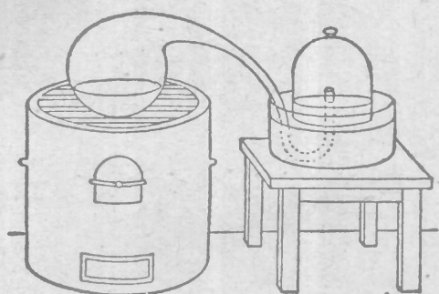
第六圖 燃燒水銀的實驗
