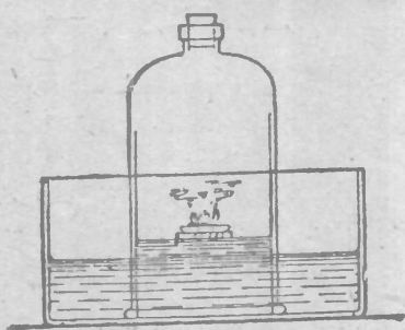
第十四圖 實驗 淡氣的性質
