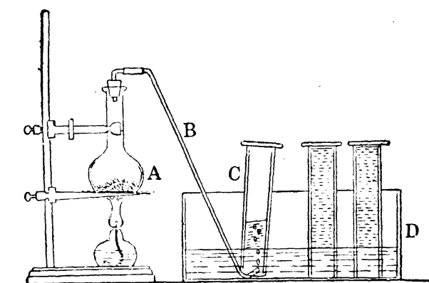
第八圖 實驗養氣的製法
