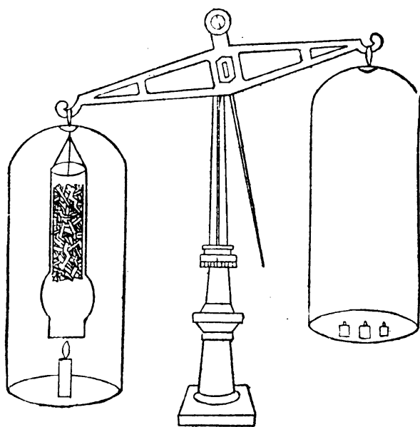
第二圖 燃燒洋燭增加重量的實驗
