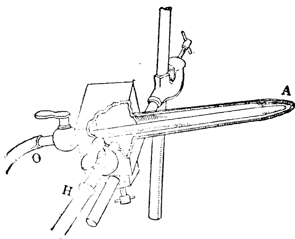
第二十四圖 輕氣和養氣混合燃 燒的器具
