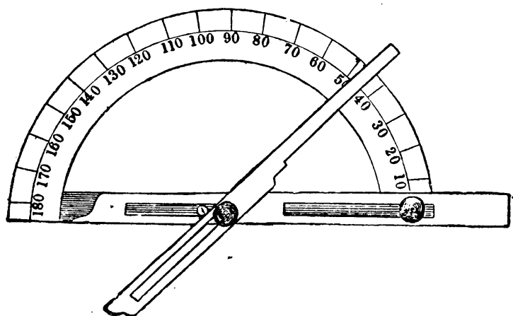
第二十八圖 測角器
