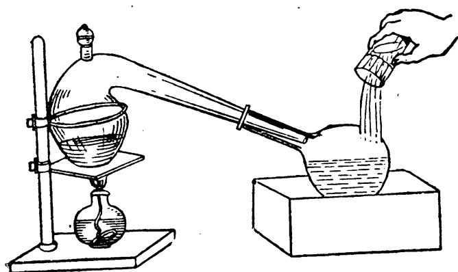
第十七圖 水的蒸餾
