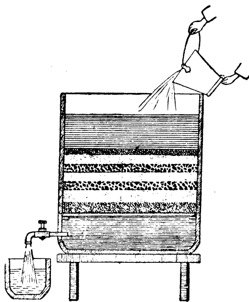
第十六圖 濾水缸
