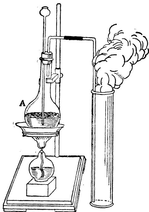
第三十一圖 氯化氫的製造
