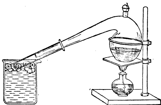
第四十九圖 硝酸的製造
