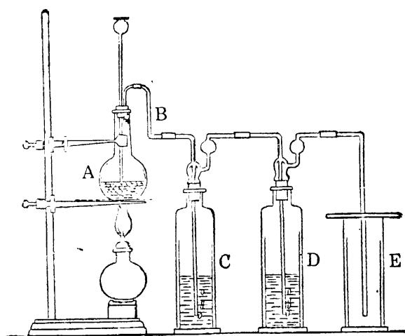
第三十五圖 綠氣的製法
