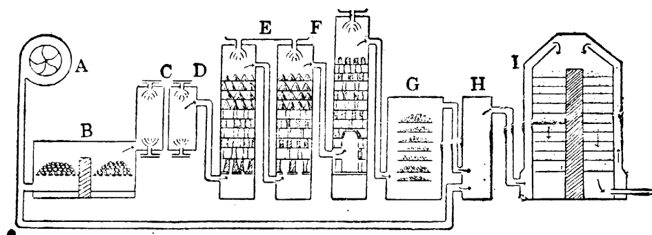
第四十七圖 接觸法
