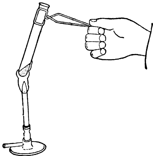
第三圖 變做化合物的實驗
