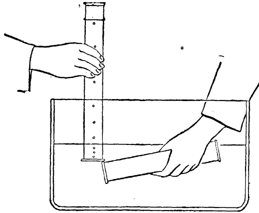
第五圖 證明空氣的存在
