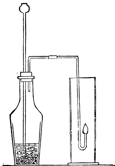
第三十六圖 輕氣在綠氣 瓶中燃燒
