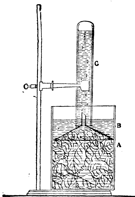
第六十圖 植物的同化作用
