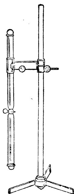
第三十四圖 綠氣與輕氣 化合的實驗
