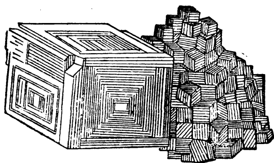
第二十七圖 食鹽的結晶
