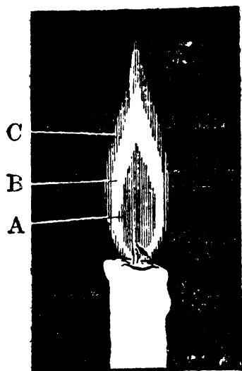
第四十四圖 火焰
