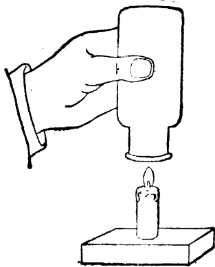
第一圖 燃點蠟燭 燭的化學變化
