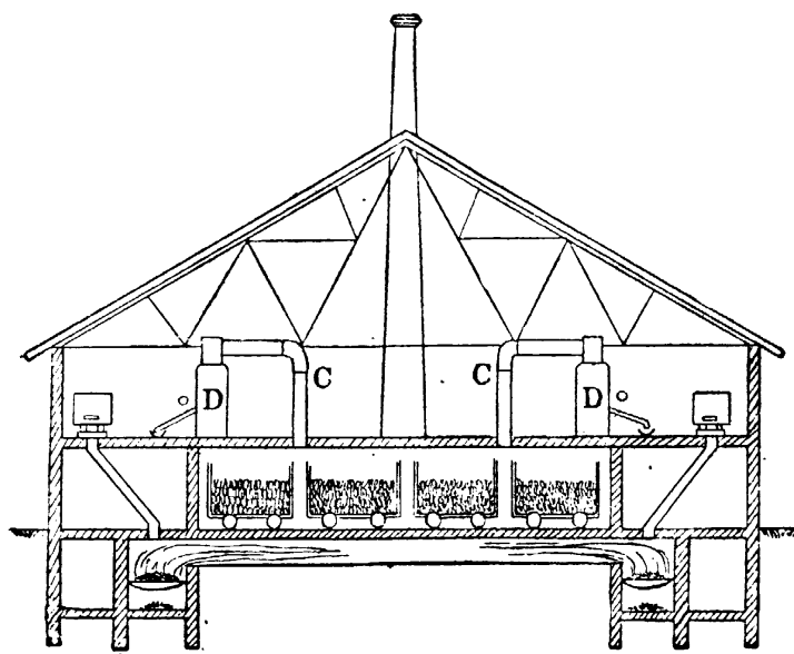
第五十五圖 木炭的製造
