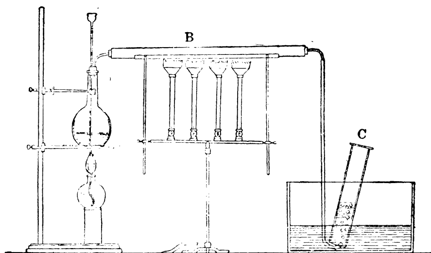
第二十一圖 製輕氣法一
