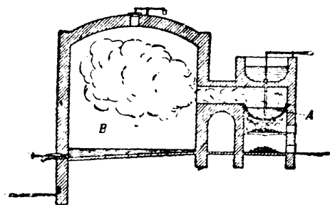
第三十八圖 硫黃的蒸餾
