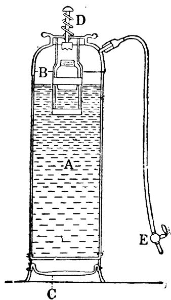
第五十八圖 滅火器
