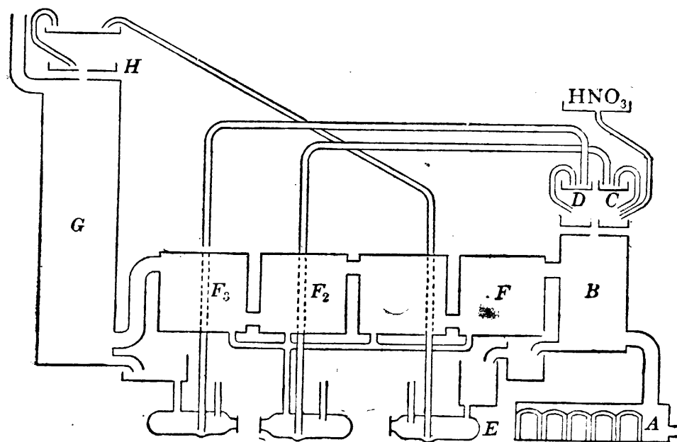
第四十八圖 鉛室法
