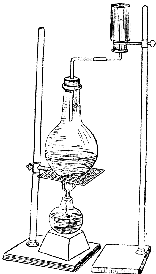
第五十一圖 氨的製造
