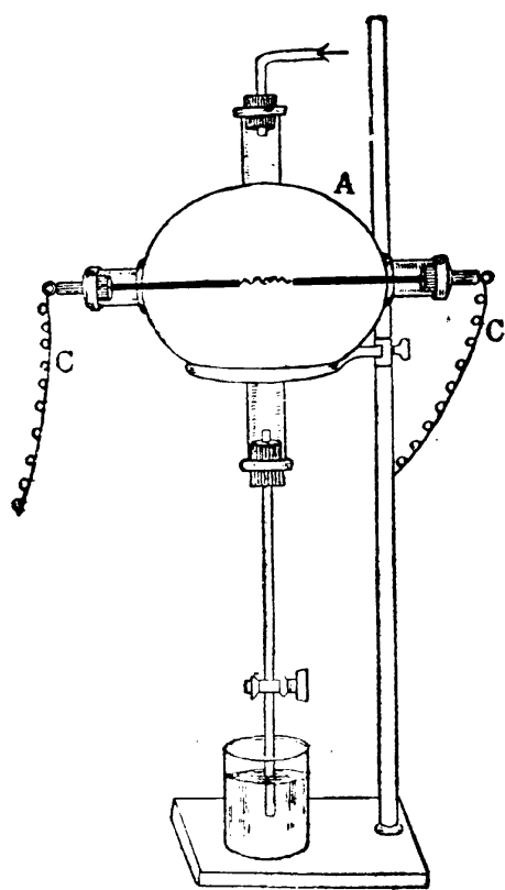
第五十圖 空氣內硝酸的生成
