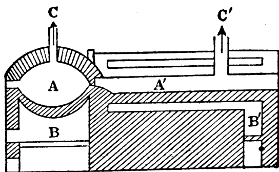
第三十二圖 工業上製造鹽酸的爐
