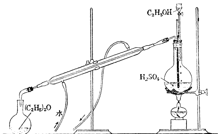
製 造 二 乙 醚
