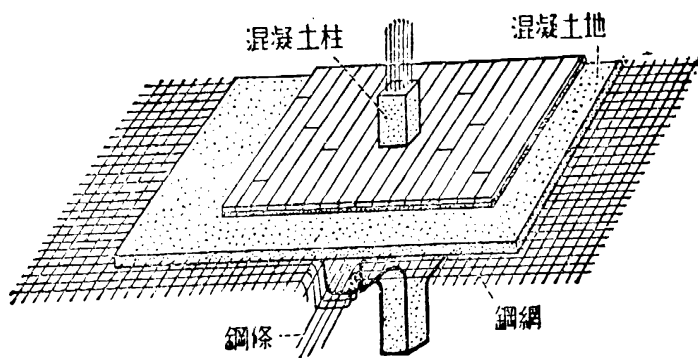
鋼骨混凝土建築的一部
