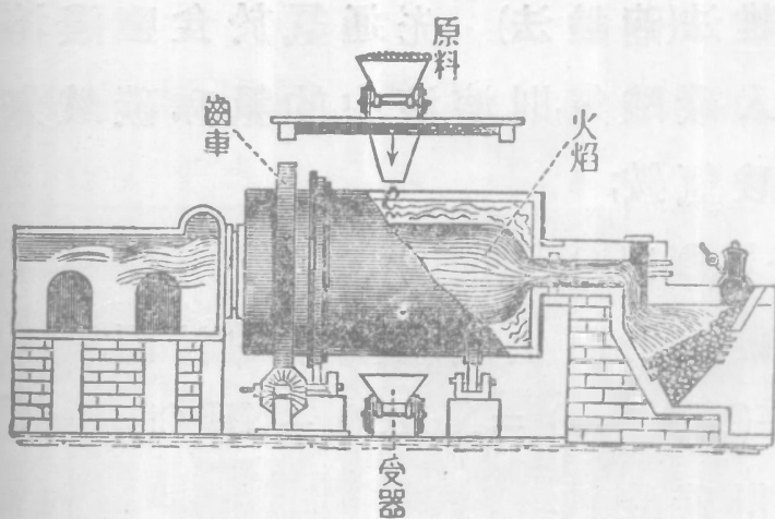
黑灰爐
