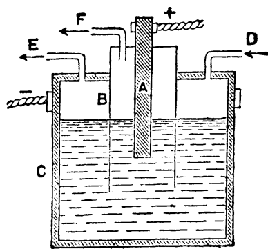
鎂 的 製 造
