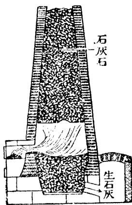
石灰窯
