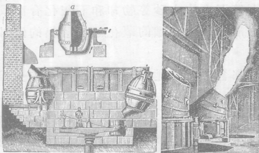
迴 轉 爐
