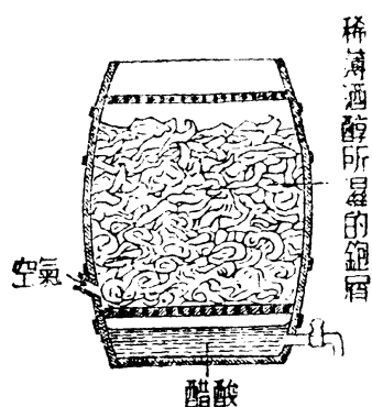
醋的製造
