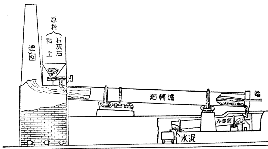
製造水泥的迴轉爐
