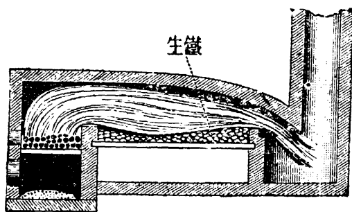
反 射 爐
