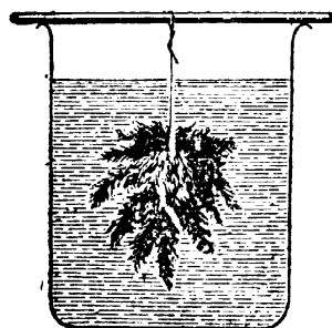
鉛 樹
