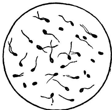
腐敗菌
