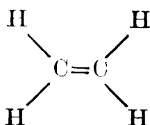
乙 烯
