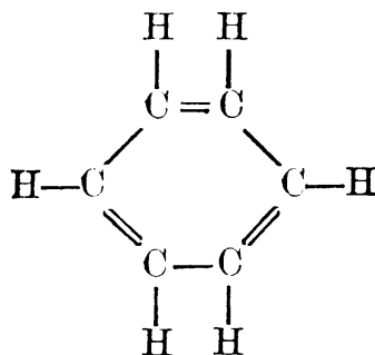
萘的構造式
