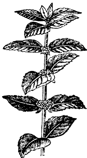
薄荷
