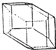
膽礬的結晶
