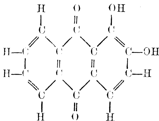
茜素的構造式
