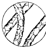
羊毛
