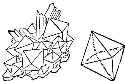
明礬的結晶
