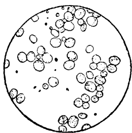
啤酒釀母
