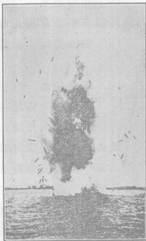
炸藥的威力
