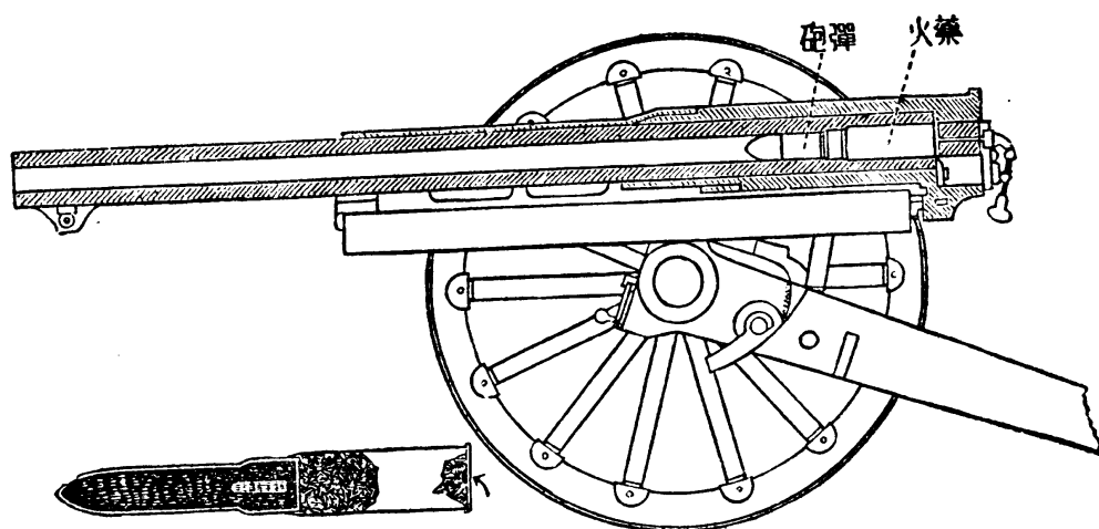
砲彈的發射
