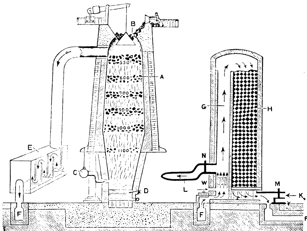
熔 鐵 爐
