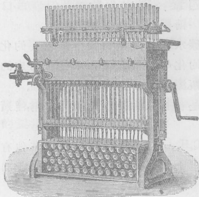
製 燭 機
