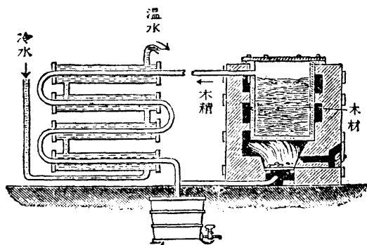
製造木精
