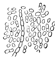
醋酸菌
