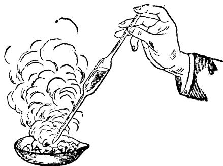
製消石灰的實驗
