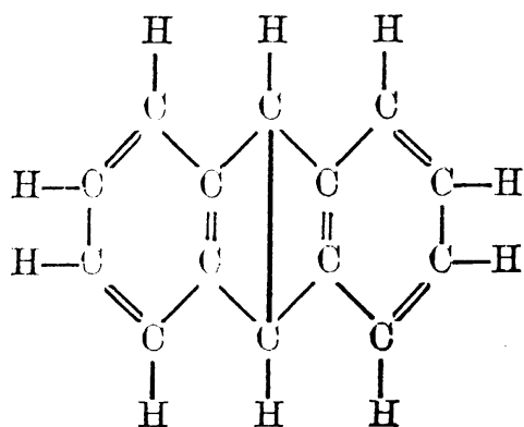
綠油腦的構造式
