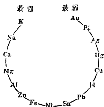
離子化傾向
