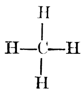
甲 烷
