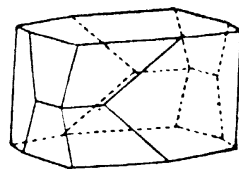
硝酸銀的結晶
