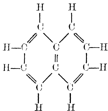
焦油腦的構造式
