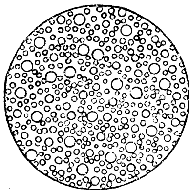
脂肪的乳狀化
