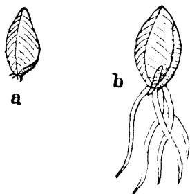
麥 芽
