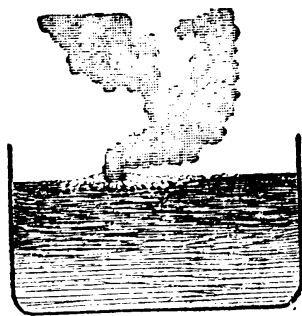
鉀分解水時輕氣自燃的情形
