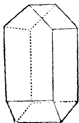
皓礬的結晶
