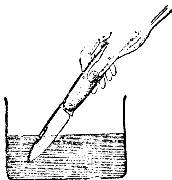
鐵比銅容易離子化
