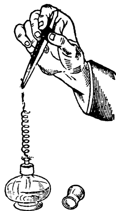
乙醛的生成
