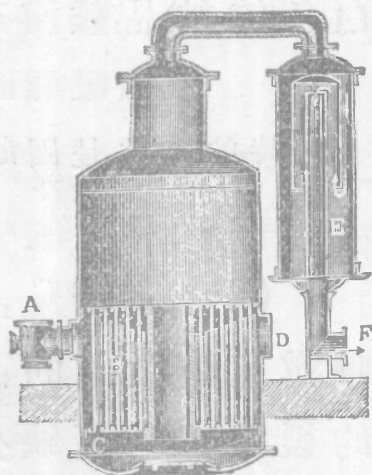
真空罐
