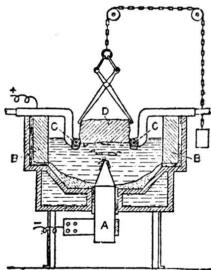
製鈣的電解裝置
