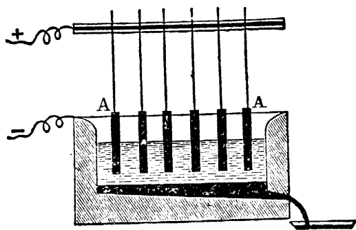
鋁的製造
