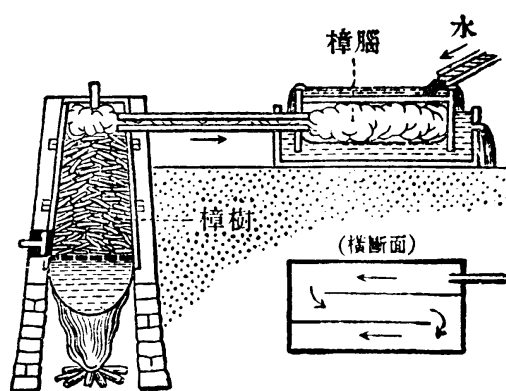
製造樟腦
