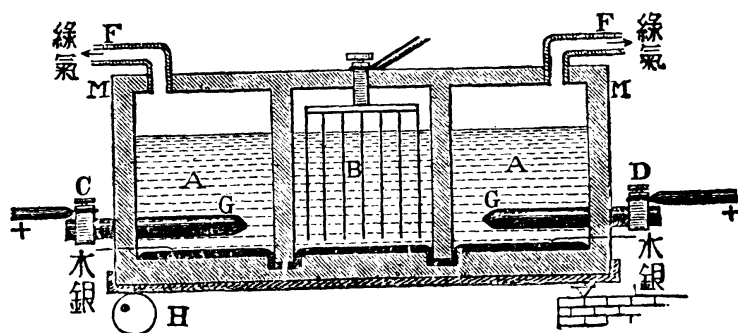
製造氫氧化鈉
