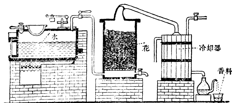
香 油 的 製 造
