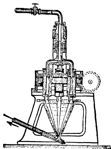
製造人造絲的機械
