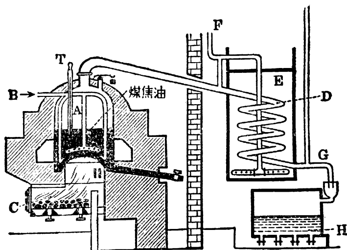
煤焦油的分溜裝置
