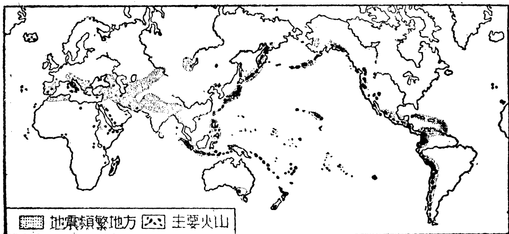
第九五圖 世界火山和地震的分佈
