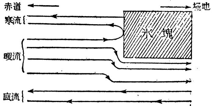
第一三五圖 海水的密度和洋流的關係
