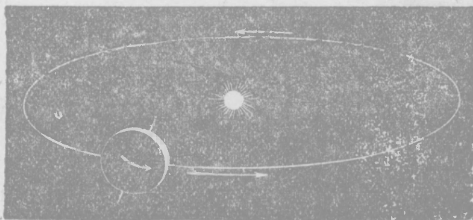
第一六圖 自轉和公轉
