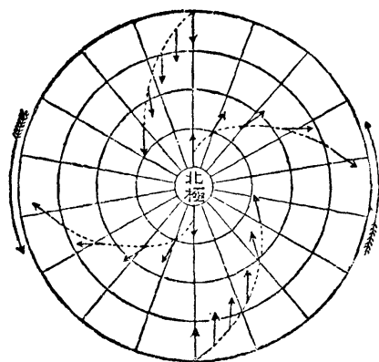
第一四七圖 北半球風向的右偏
