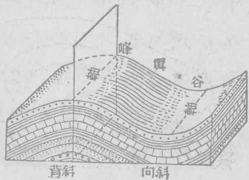
第一〇五圖 褶曲部份的名稱
