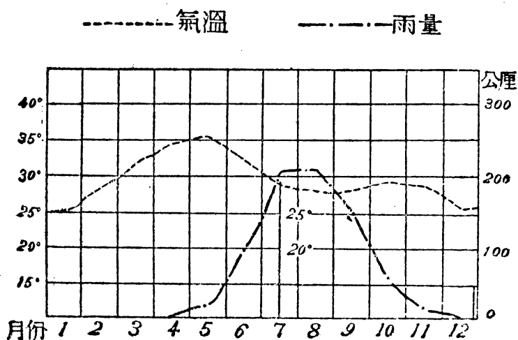
第一五八圖 卡耶斯的氣候圖表
