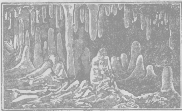
第三九圖 石灰洞
