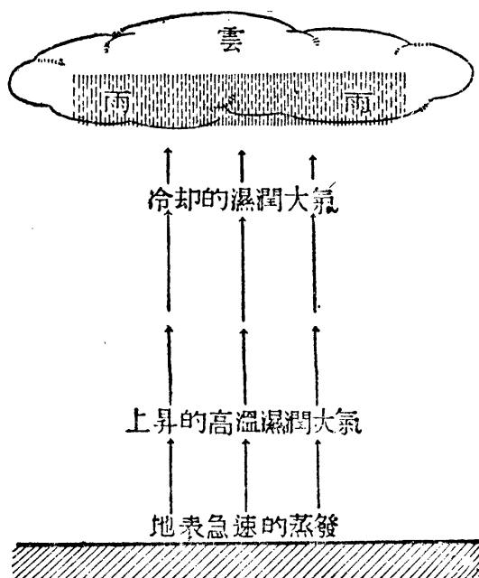
第一五二圖 對流性降雨
