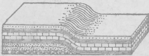
第一〇三圖 拗褶
