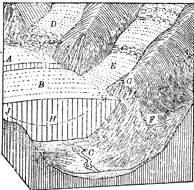
第七〇圖 懸谷的形成
