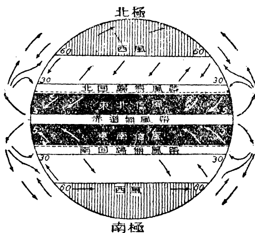
第一五〇圖 地球上氣流的循環
