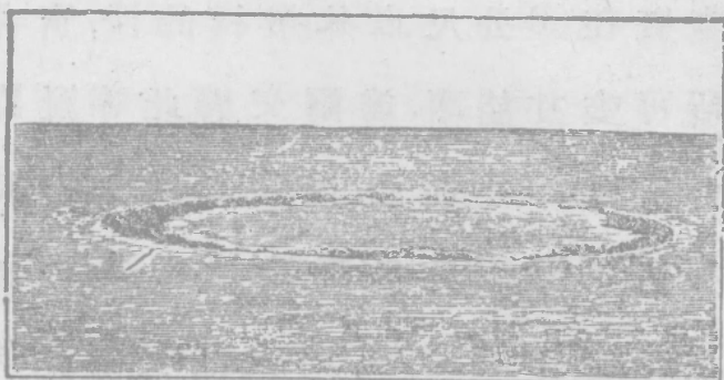
第八二圖 環礁
