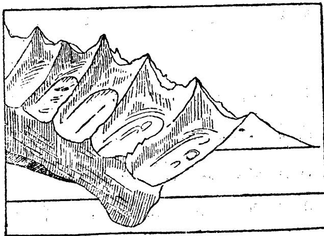
第六九圖 冰河谷源的圈谷
