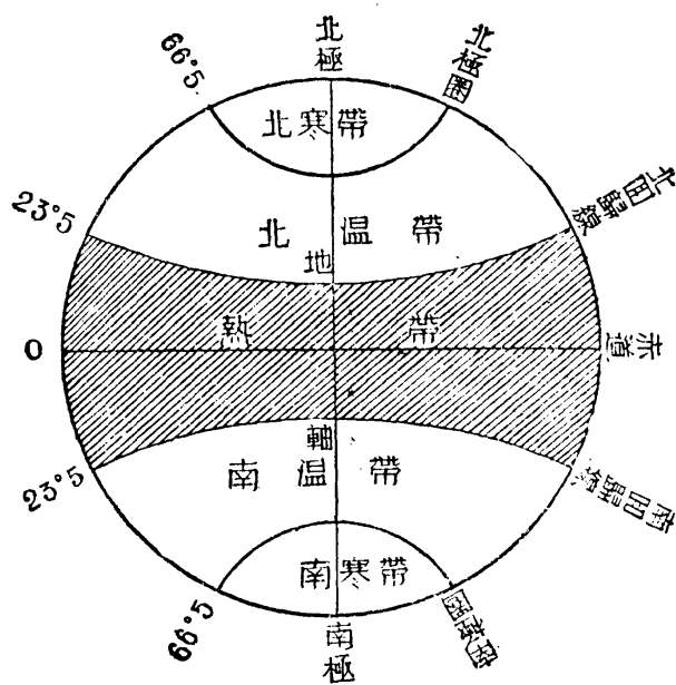
第二〇圖 五帶
