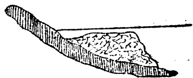
第七八圖 裾礁
