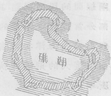
第八一圖 環礁
