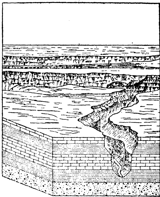
第一一四圖 亞利桑那的侵蝕谷
