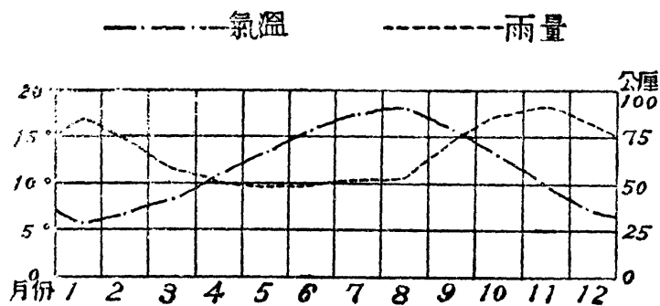
第一六四圖 布勒斯特的氣候圖表
