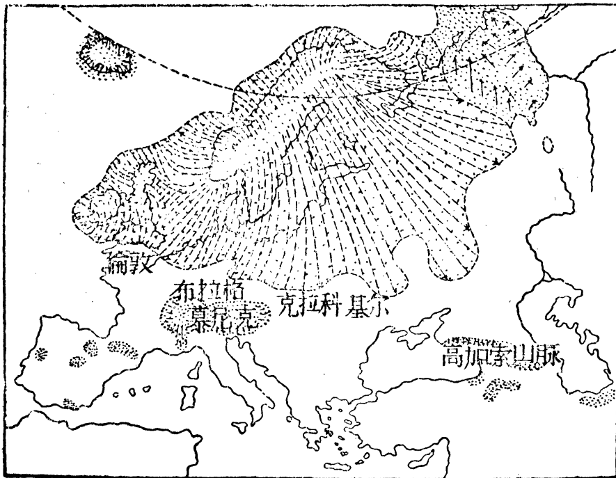
第七二圖 歐洲冰期內陸冰的被覆地域
