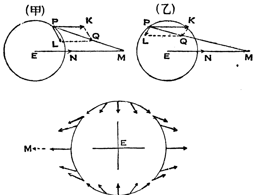
第一三二圖 潮汐的成因
