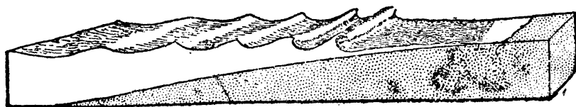
第一三一圖 磯波的斷面
