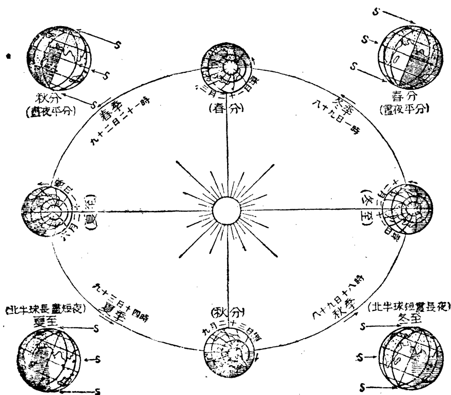
第一九圖 四季循環圖
