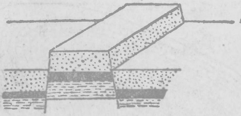
第一〇二圖 地壘
