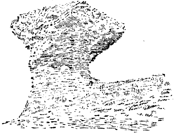
第二八圖 覃狀石
