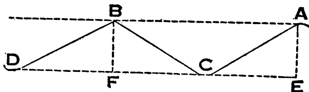
第一二九圖 波的運動
