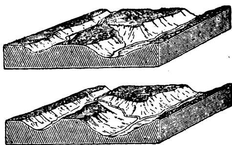
第一一五圖 河川的爭奪
