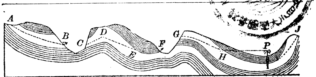
第三七圖 自流井 (P 即自流井)
