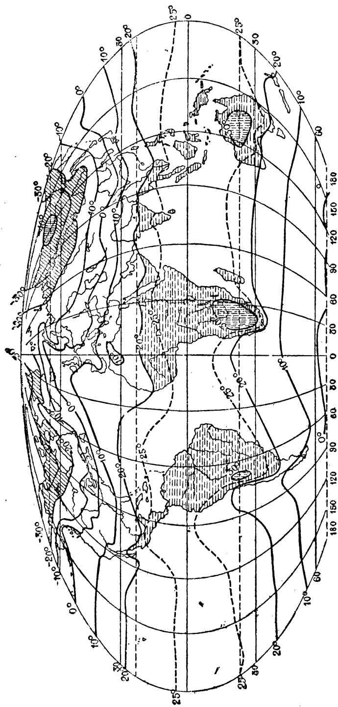
第一四三圖 一月等溫線分佈圖
