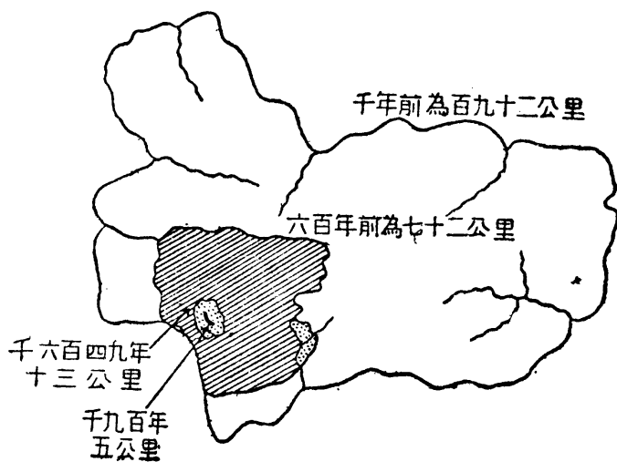
第五五圖 黑里哥蘭島可驚的海蝕
