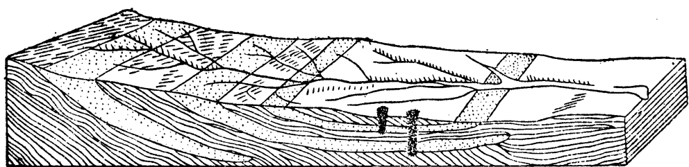
第三六圖 地 下 水
