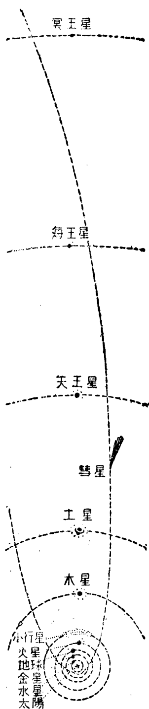
第一圖 太陽系
