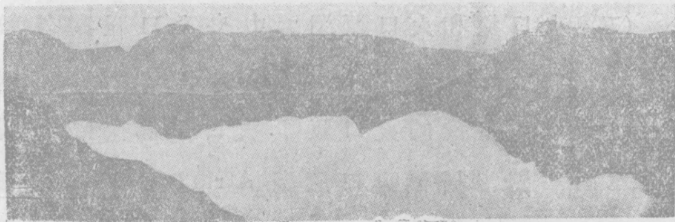
第八八圖 長白山的天池
