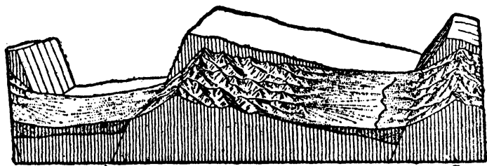
第一一三圖 斷層山岳和侵蝕
