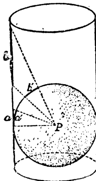
第二三圖 各種投影圖法
