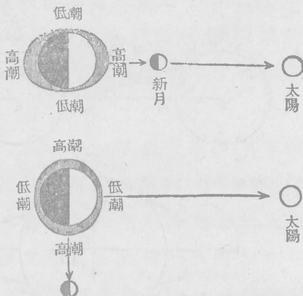
第一三三圖 大潮和小潮
