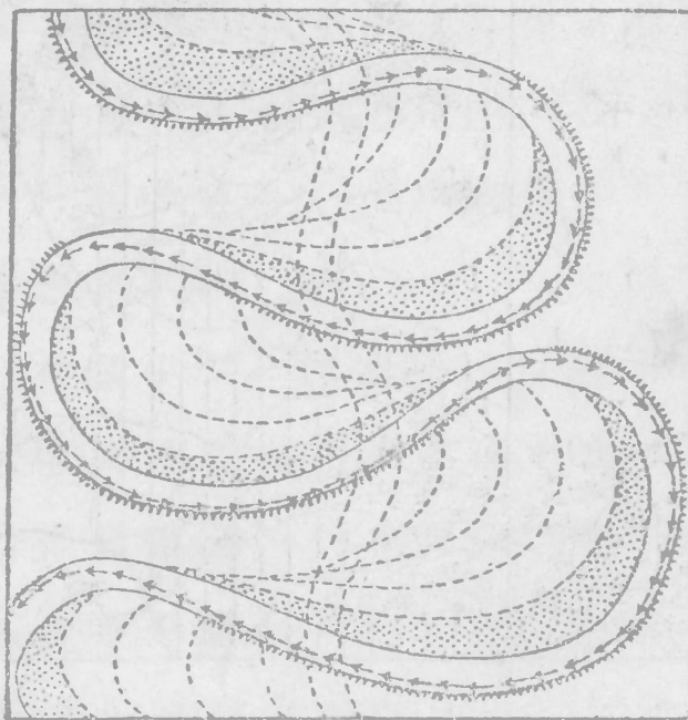
第五一圖 蛇曲的發達
