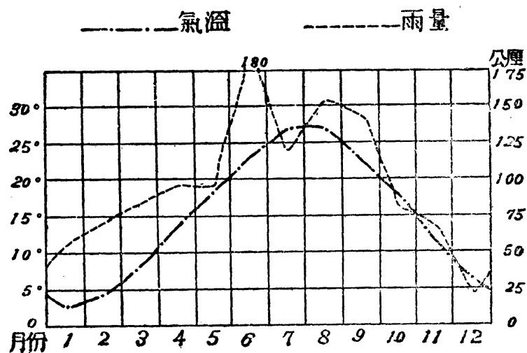
第一六一圖 上海的氣候圖表
