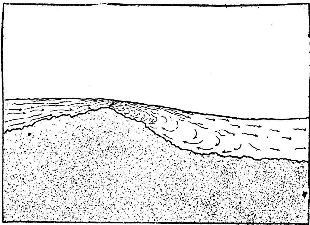
第四四圖 長江激流的成因(甲)
