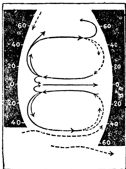
第一三六圖 洋流的二大環流
