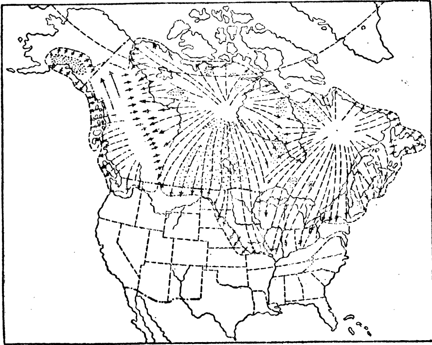
第七三圖 北美冰期內陸冰的被覆地域
