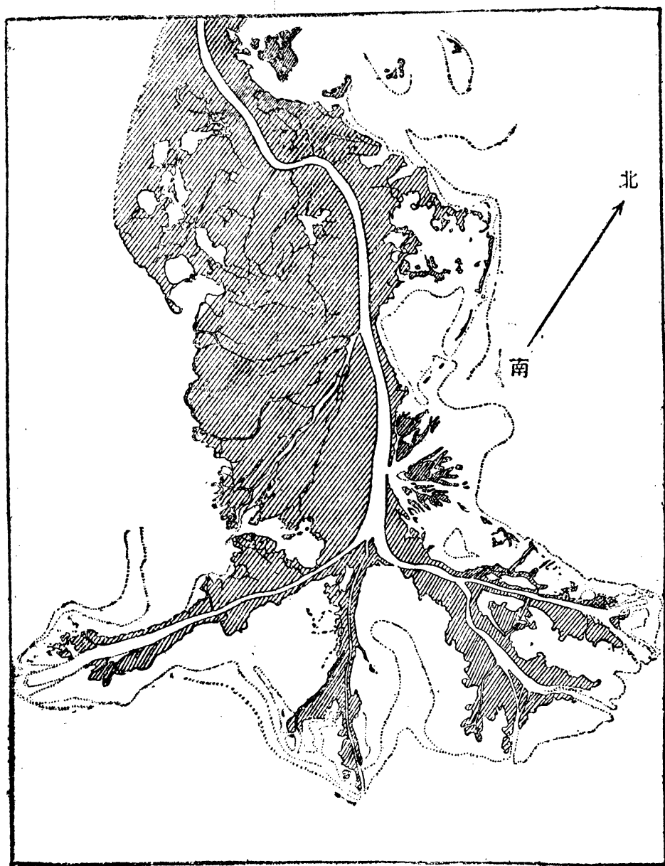
第五四圖 密士失必河三角洲
