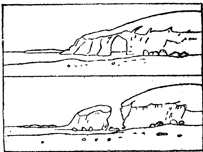
第五六圖 陸橋與顯礁
