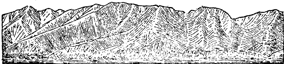
第六六圖 挽捩作用所成的岩崖
