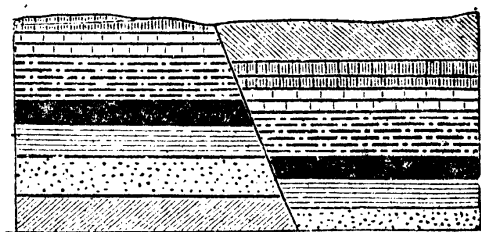
第九九圖 斷層
