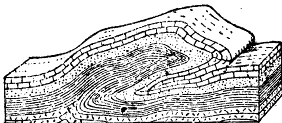
第一〇七圖 偃臥褶曲
