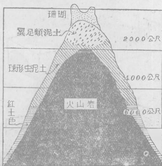
第八四圖 墨累氏的隆起說圖解
