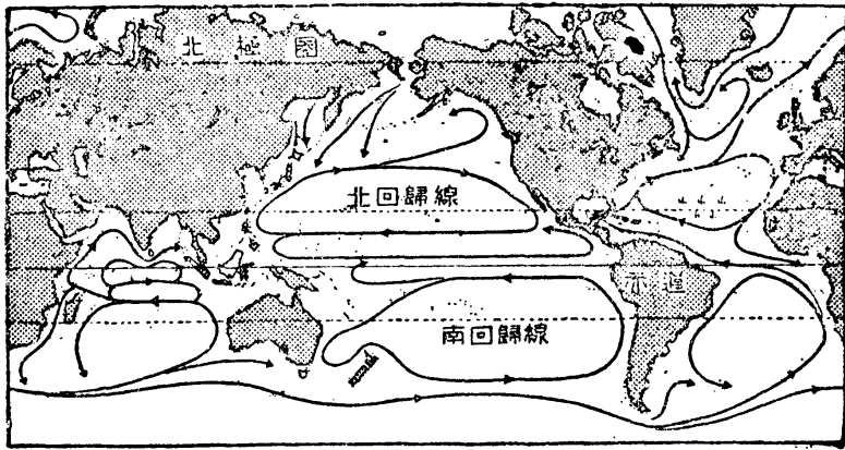
第一三八圖 主要洋流的方向
