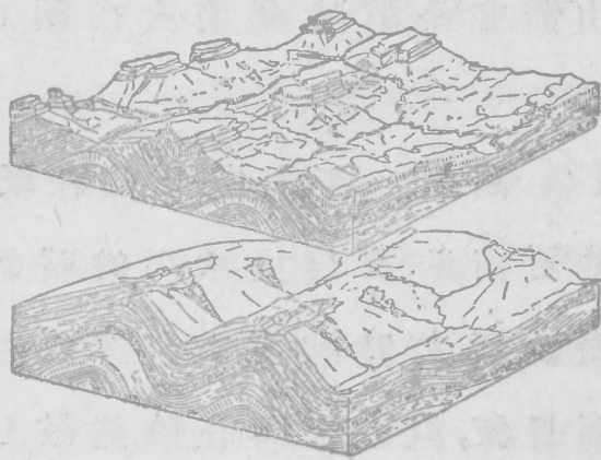
第一一二圖 褶曲山地地形的演化
