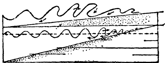
第一三〇圖 磯波
