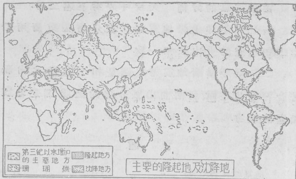
第九六圖 世界汀線變動圖
