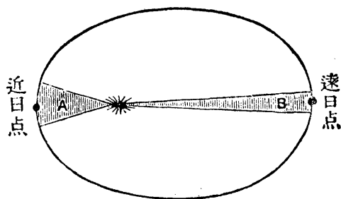
第一八圖 近日點和遠日點
