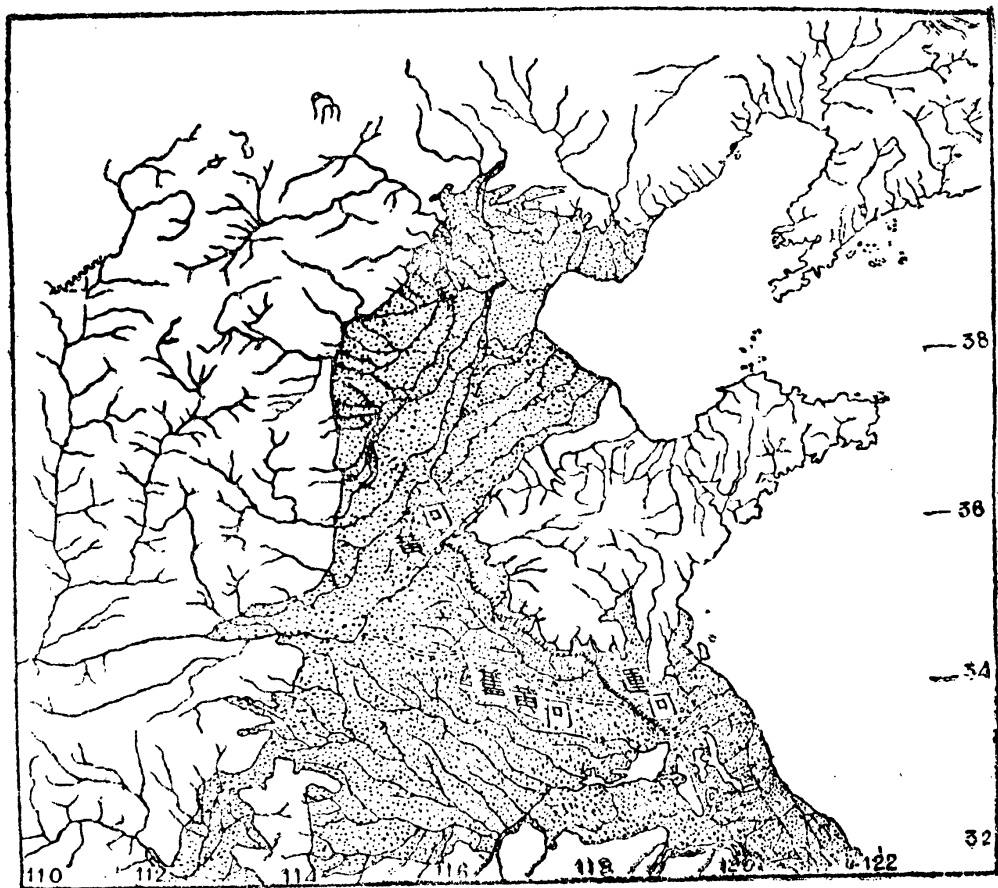
第五二圖 黄河的遷徙
