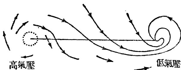
第一四六圖 北半球高低氣壓的偏向
