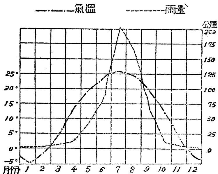
第一六二圖 北平的氣候圖表
