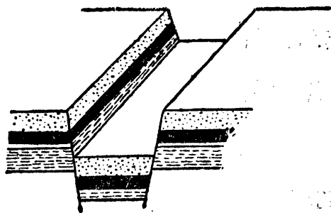
第一〇一圖 地塹
