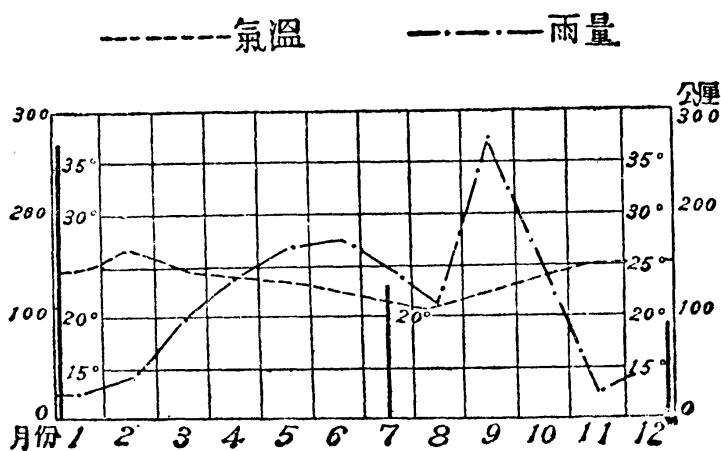
第一五七圖 俾斯麥堡的氣候圖表
