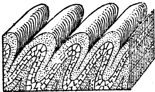
第一〇八圖 等斜褶曲
