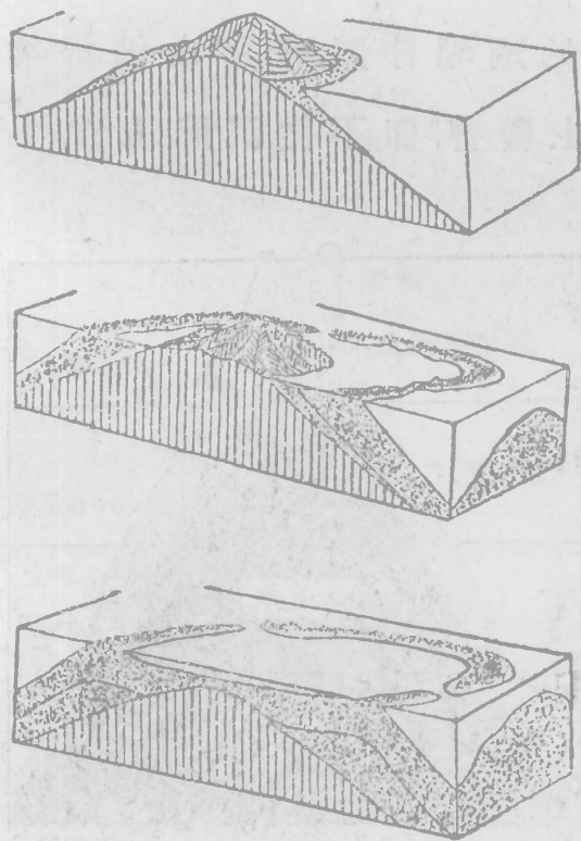
第八三圖 達爾文氏的沈降說圖解
