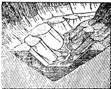
第一一七圖 河成階段
