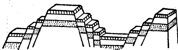
第一〇〇圖 階狀斷層和地塹地壘
