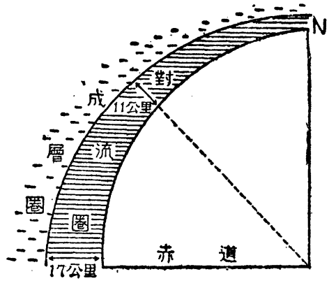
第一三九圖 成層圈和對流圈
