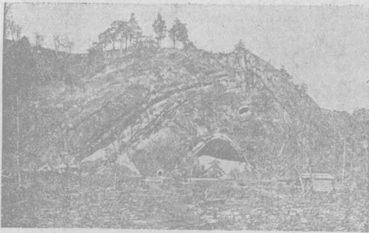
第一〇三圖 拗褶
