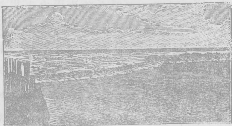
第一三四圖 錢塘潮
