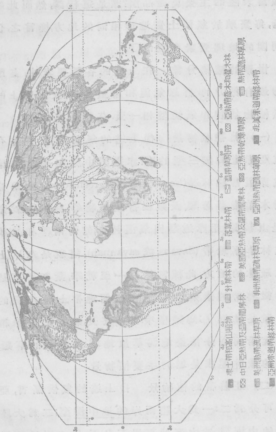
第一六八圖 世界植物分佈圖
