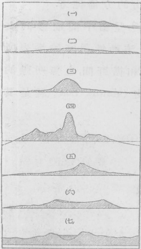
第九一圖 火山的形態
