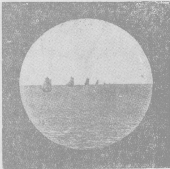
第八圖 哥白尼氏的發見
