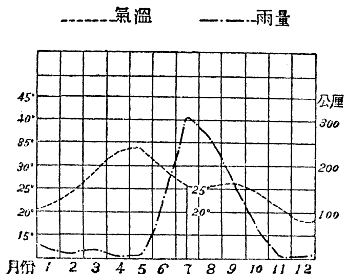
第一六〇圖 那哥不爾的氣候圖表
