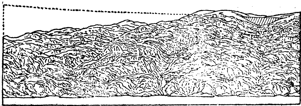
第六五圖 冰河研磨所成的地形
