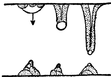
第四〇圖 點滴石的生成
