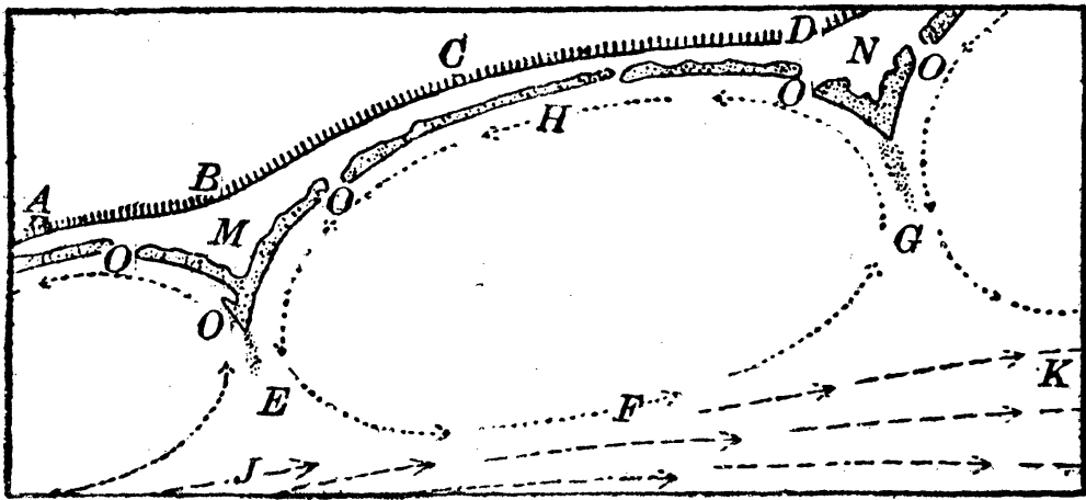
第六〇圖 美國卡羅來納州的遠岸洲
