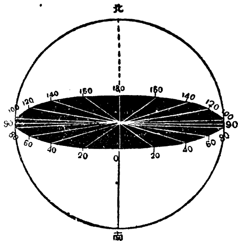
第一一圖 經度
