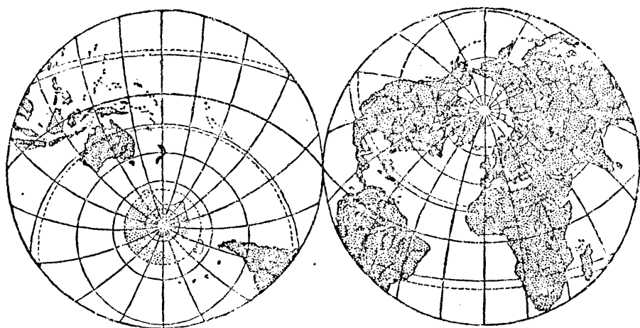
第二六圖 水半球和陸半球
