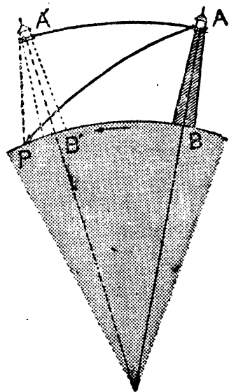
第一七圖 落體的東偏
