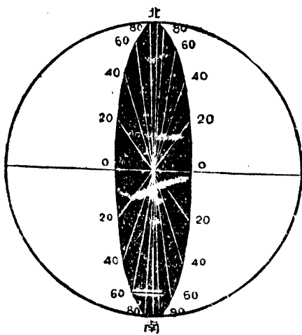
第一二圖 緯度
