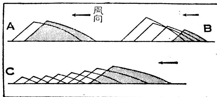
第三二圖 砂丘的移動
