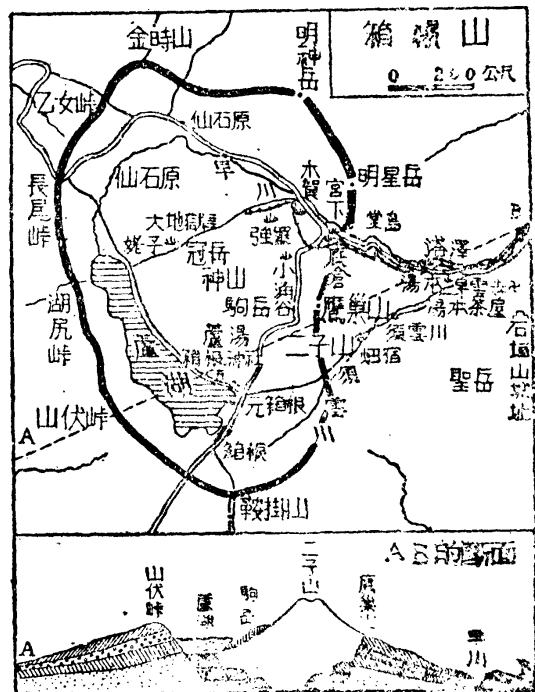
第八七圖 複火山的箱根
