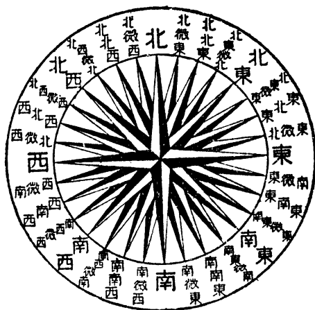
第一三圖 方位的名稱
