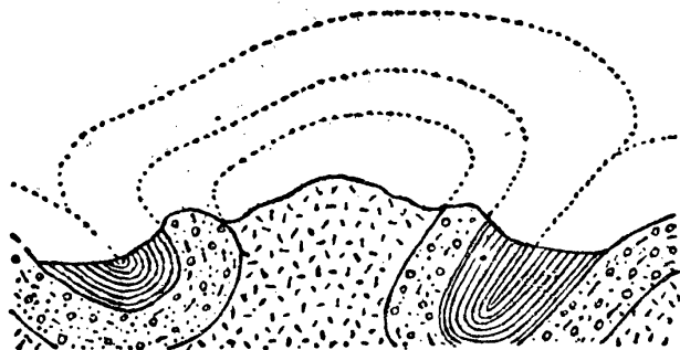
第一〇九圖 扇形褶曲
