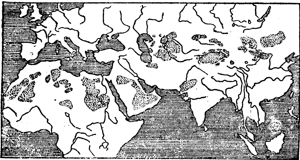
第三四圖 世界沙漠(多砂丘)的分佈地
