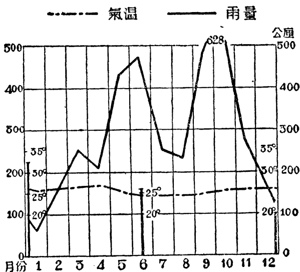
第一五六圖 阿卡撒的氣候圖表
