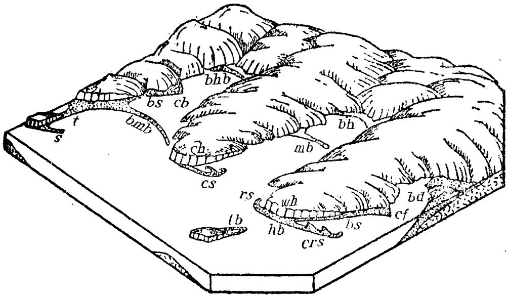
第五八圖 海岸堆積地形圖
