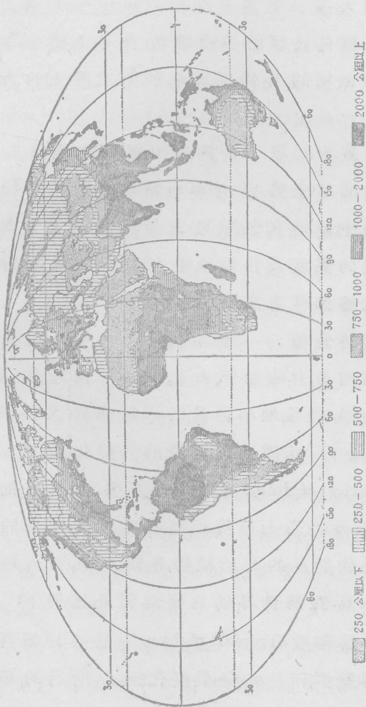
第一五四圖 年平均雨量分佈圖
