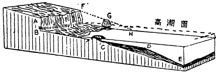
第五七圖 海蝕地形圖
