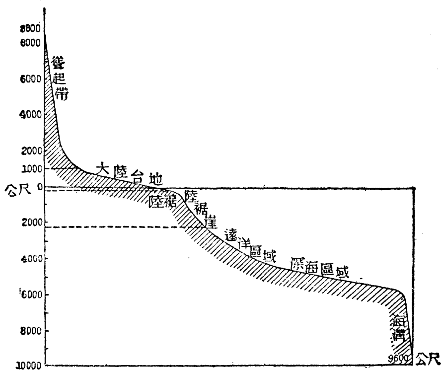
第一一八圖 海底的地形
