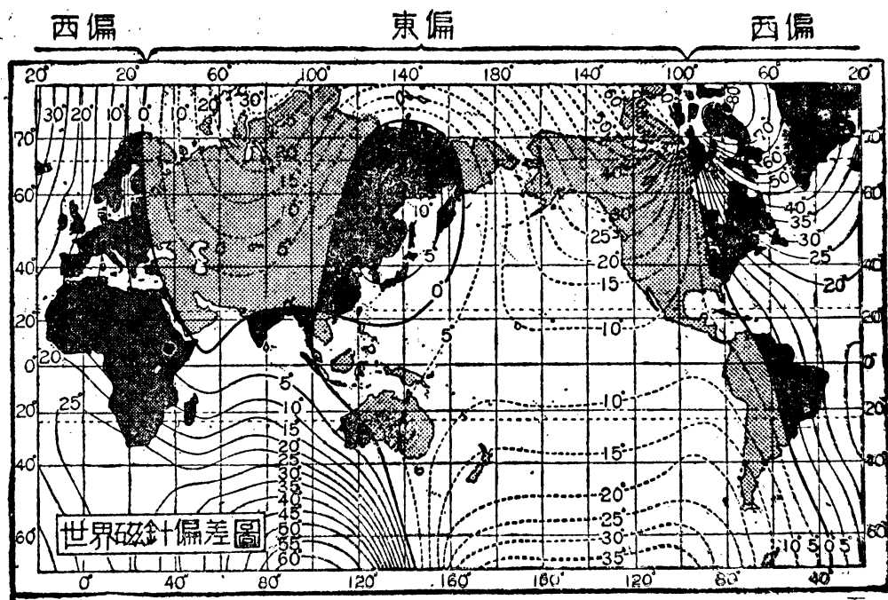
第一四圖 世界磁針偏差圖
