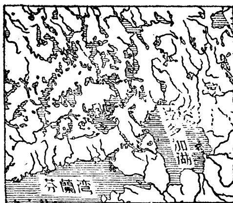
第七一圖 芬蘭的湖沼地方
