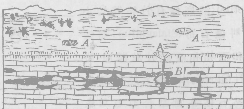
第三八圖 石灰岩地的斷面
