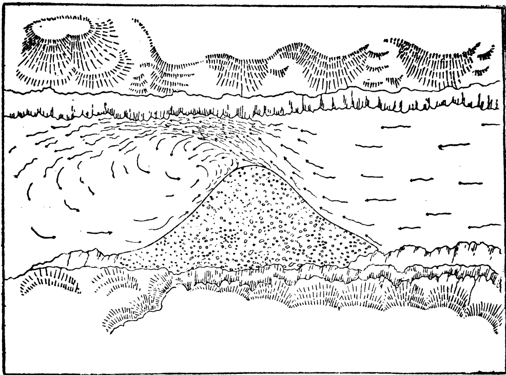
第四六圖 長江激流的成因(丙)
