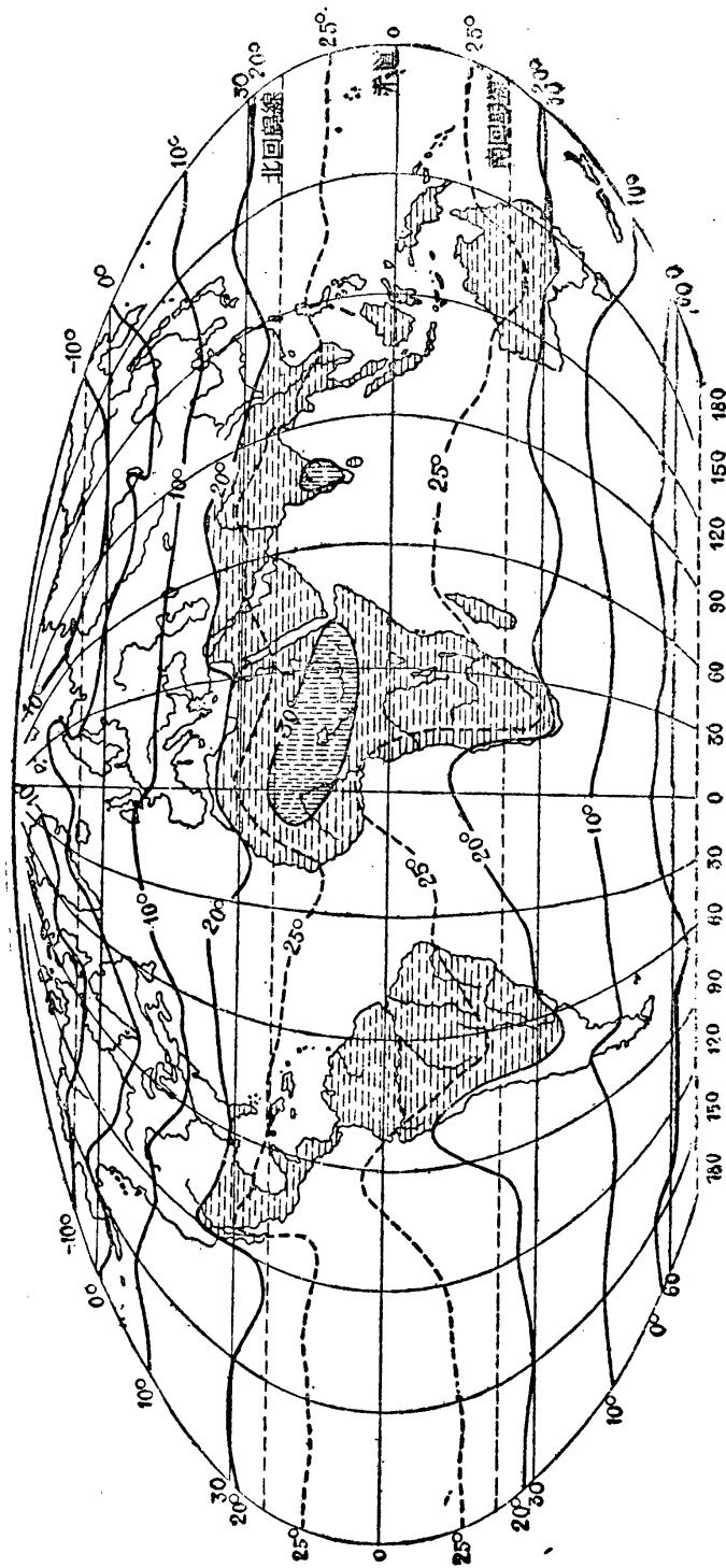
第一一四圖 年平均等溫線分佈圖
