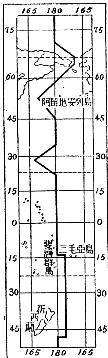
第二二圖 日期變更線
