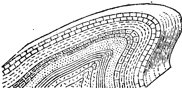
第一〇六圖 過褶曲
