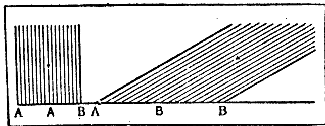
第一四一圖 太陽光的斜射和直射
