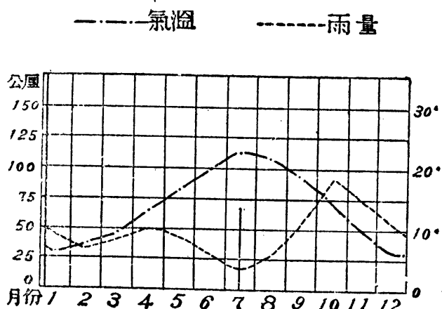
第一六三圖 馬賽的氣候圖表
