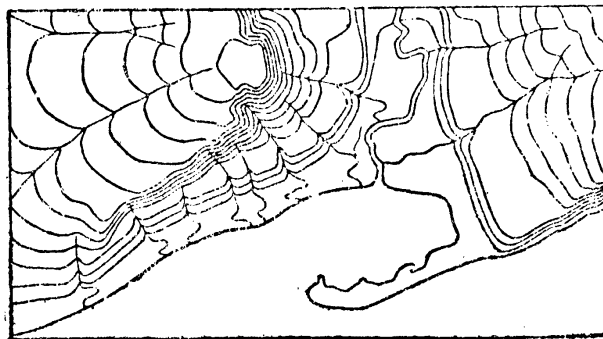
第二四圖 地形圖 上. 地塊圖 中. 暈滃圖 下. 等高線圖
