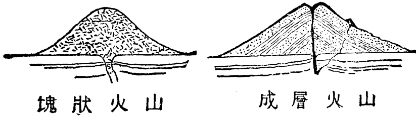
第八六圖 塊狀火山和成層火山
