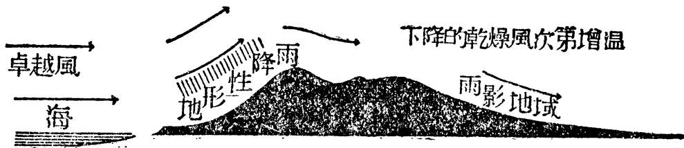
第一五三圖 地形性降雨
