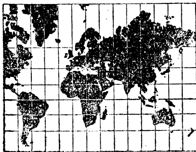
第二三圖 各種投影圖法
