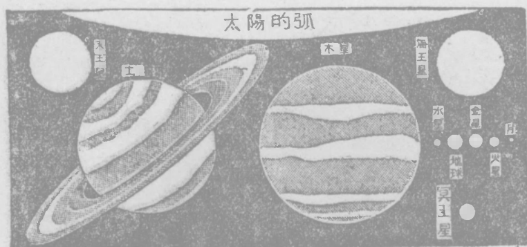
第二圖 太陽和各大行星大小的比較
