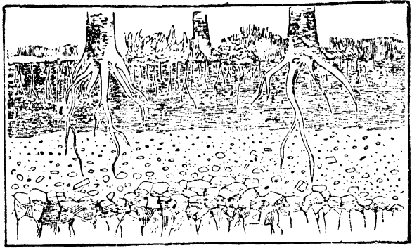
第七四圖 植物根的作用
